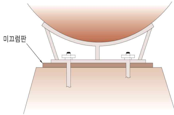
그림 2.2.3.5 미끄럼판의 설치 방법
