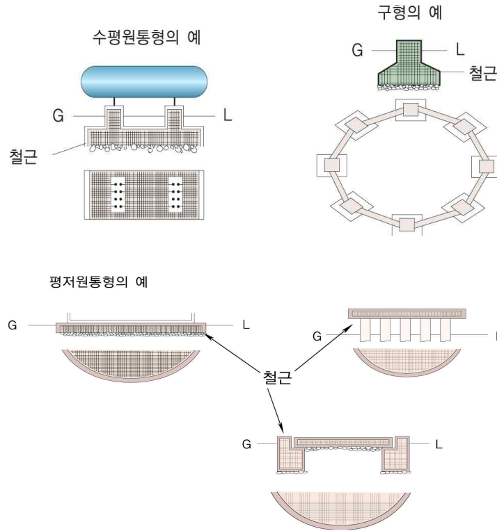
그림 2.2.2.3 저장탱크의 수평 기초면
