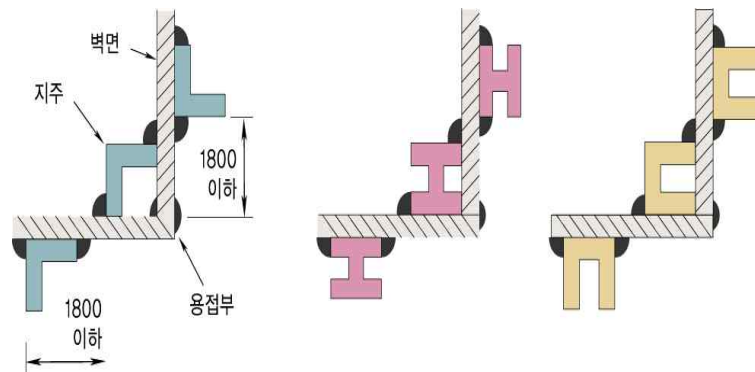
그림 2.8.2.3.4 지주의 설치 방법
