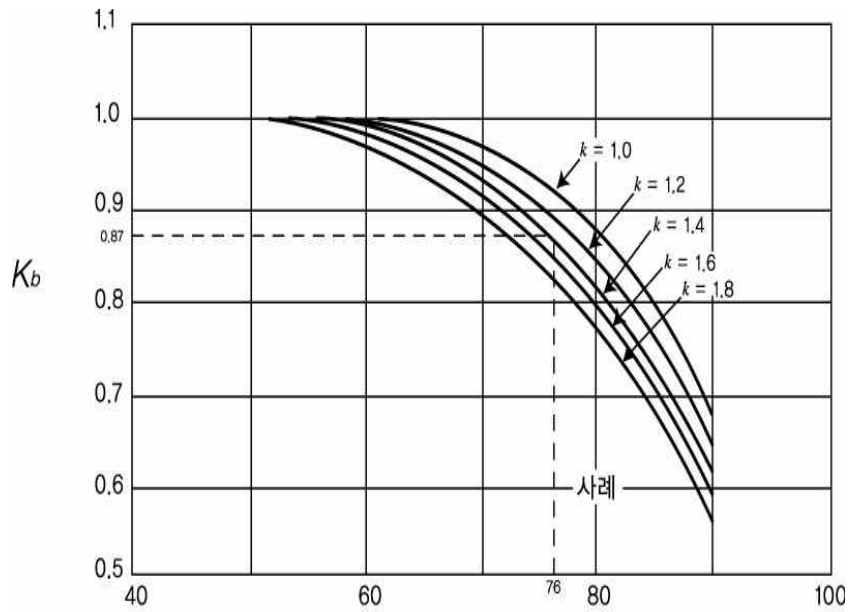
그림 2.7.1.4.1② 밸런스 벨로즈형 안전밸브 배압보정계수
