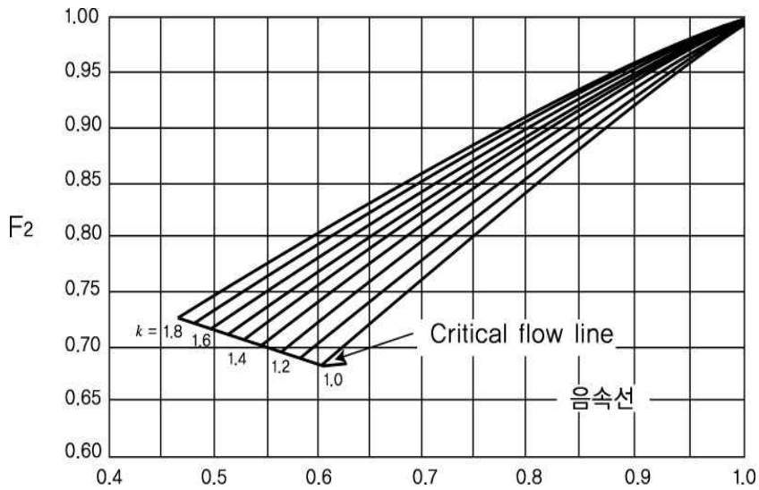
그림 2.7.1.4.1④ 압축계수
