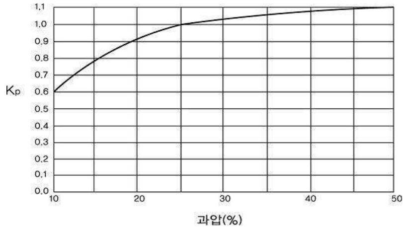
그림 2.6.1.4⑧ 과압보정계수
