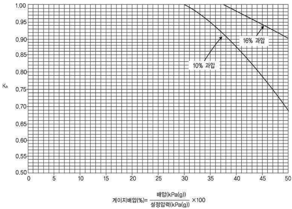
그림 2.6.1.4② 밸런스 벨로즈형 안전밸브 배압보정계수
