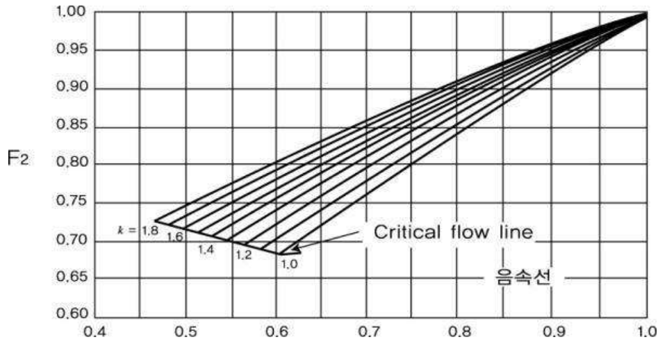
그림 2.6.1.4⑤ 이음속계수
