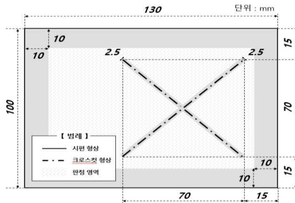
그림 C4.(2) 도장을 한 금속재료 시험편의 크로스컷 형상 및 판정 영역
