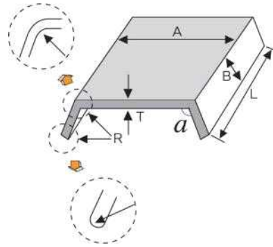
그림 2.5.4.2.6 보호판의 치수
