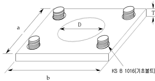
그림 2.3.3.4(6-4-2) 강관제 보호대의 받침대 설치 방법
