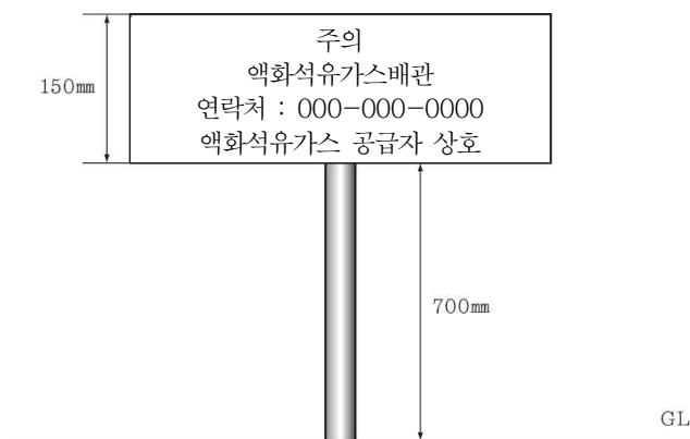
그림 2.5.10.3.3(4) 표지판의 치수 및 표기방법의 예시
