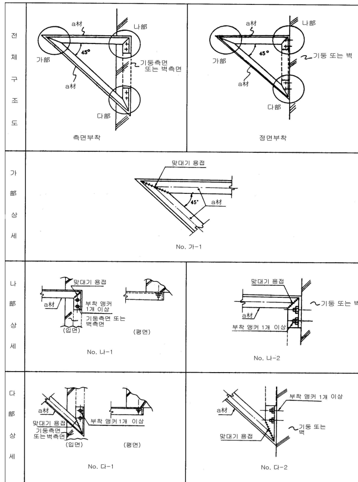
그림 F9.4 황지관 내진지지구 상세도 및 조립요령
