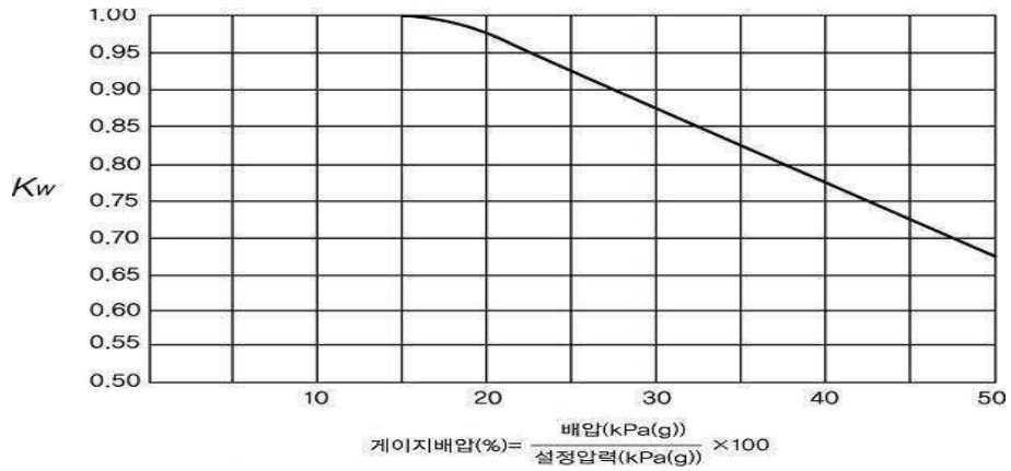
그림 2.8.1.4.1(2)⑥ 벨런스벨로우즈형 안전밸브 배압보정계수
