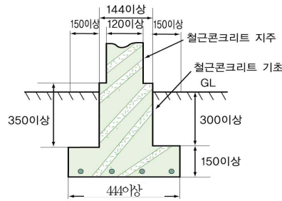
그림 2.9.2.1 철근콘크리트제 방호벽 설치예 <개정 23. 7. 3.>
