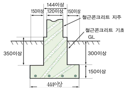
그림 2.9.2.1 철근콘크리트제 방호벽 설치예 <개정 23. 7. 3.>
