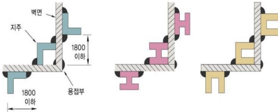
그림 2.9.2.3.4 지주의 설치방법
