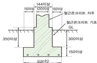
그림 2.9.2.1 철근콘크리트제 방호벽 설치에 <개정 23. 7. 3.>
