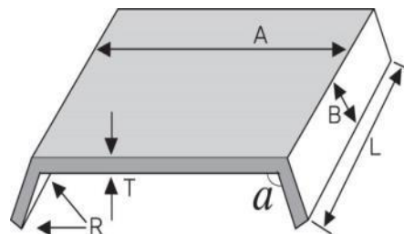
그림 2.5.7.2.3 보호판의 치수 측정
