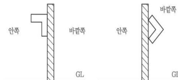
그림 2.9.2.3.2 강판제방호벽의 앵글강 보강
