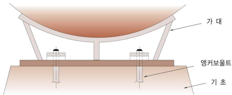
그림 2.2.3.4 앵커볼트의 고정 방법
