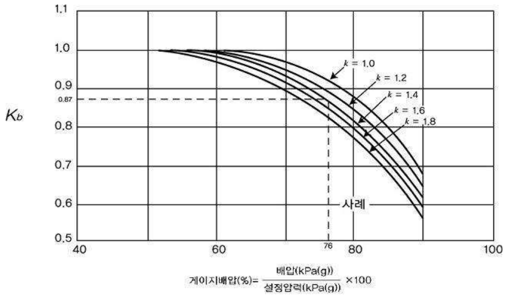
그림 2.6.1.4② 밸런스 벨로즈형 안전밸브 배압보정계수
