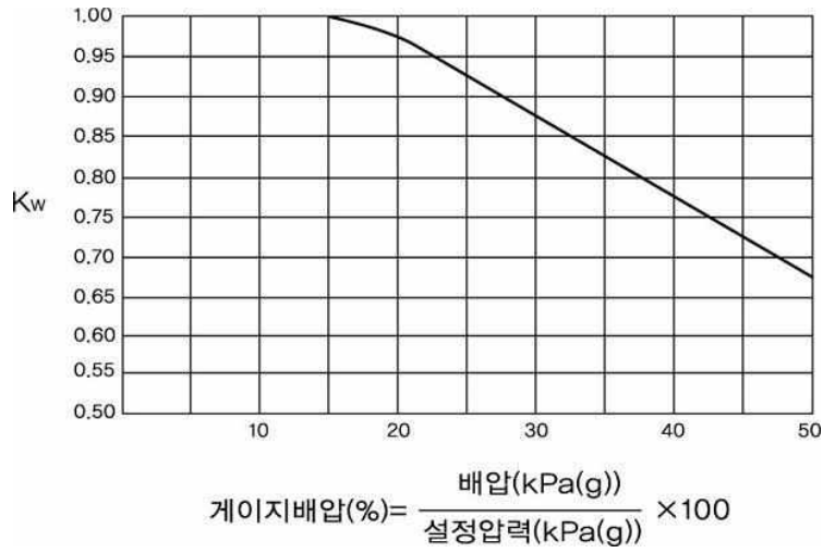
그림 2.6.1.4⑥ 벨런스 벨로즈형 안전밸브 배압보정계수
