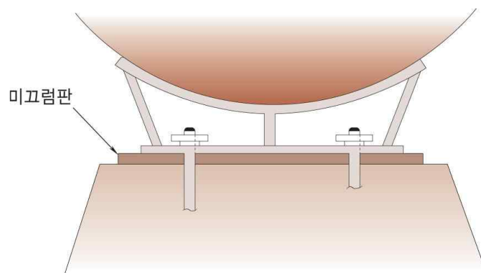
그림 2.2.3.5.3 미끄럼판의 설치 방법
