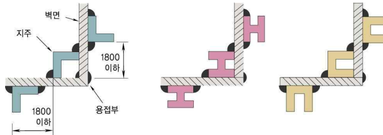
그림 2.7.2.3.4 지주의 설치 방법
