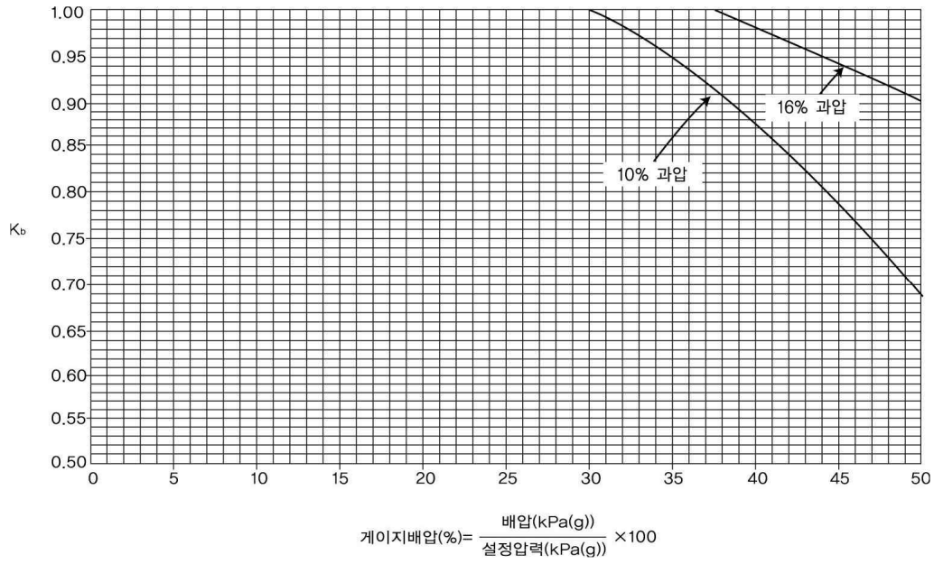
그림 2.6.1.4② 밸런스 벨로즈형 안전밸브 배압보정계수
