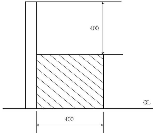
그림 2.7.2.2.3 보조벽의 높이
