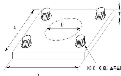
그림 2.4.4.2.1(6-4-2) 강관제 보호대의 받침대 설치 방법
