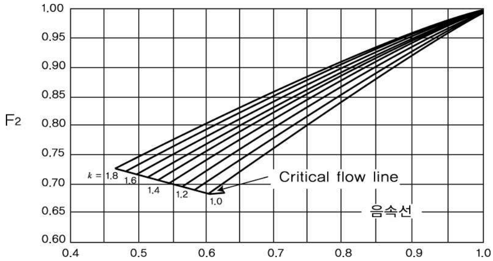
그림 2.6.1.4⑤ 아음속계수
