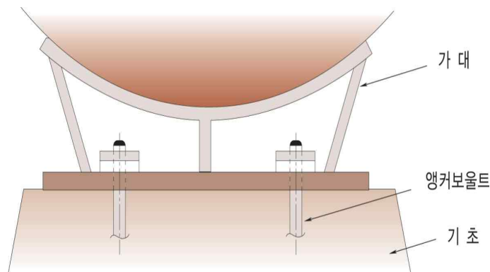
그림 2.2.3.4 앵커볼트의 고정방법
