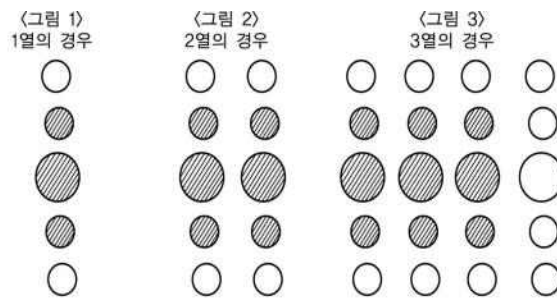
그림 2.7.9.1.3 온도상승방지설비 능력산정기준
