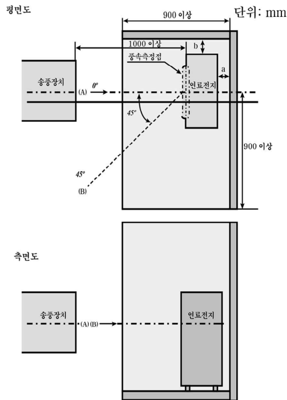
그림 C4 유증시험장치
