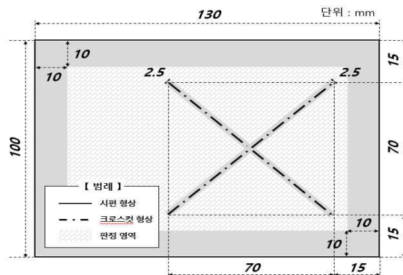
그림 C1.(2) 도장을 한 금속재료 시험편의 크로스컷 형상 및 판정 영역
