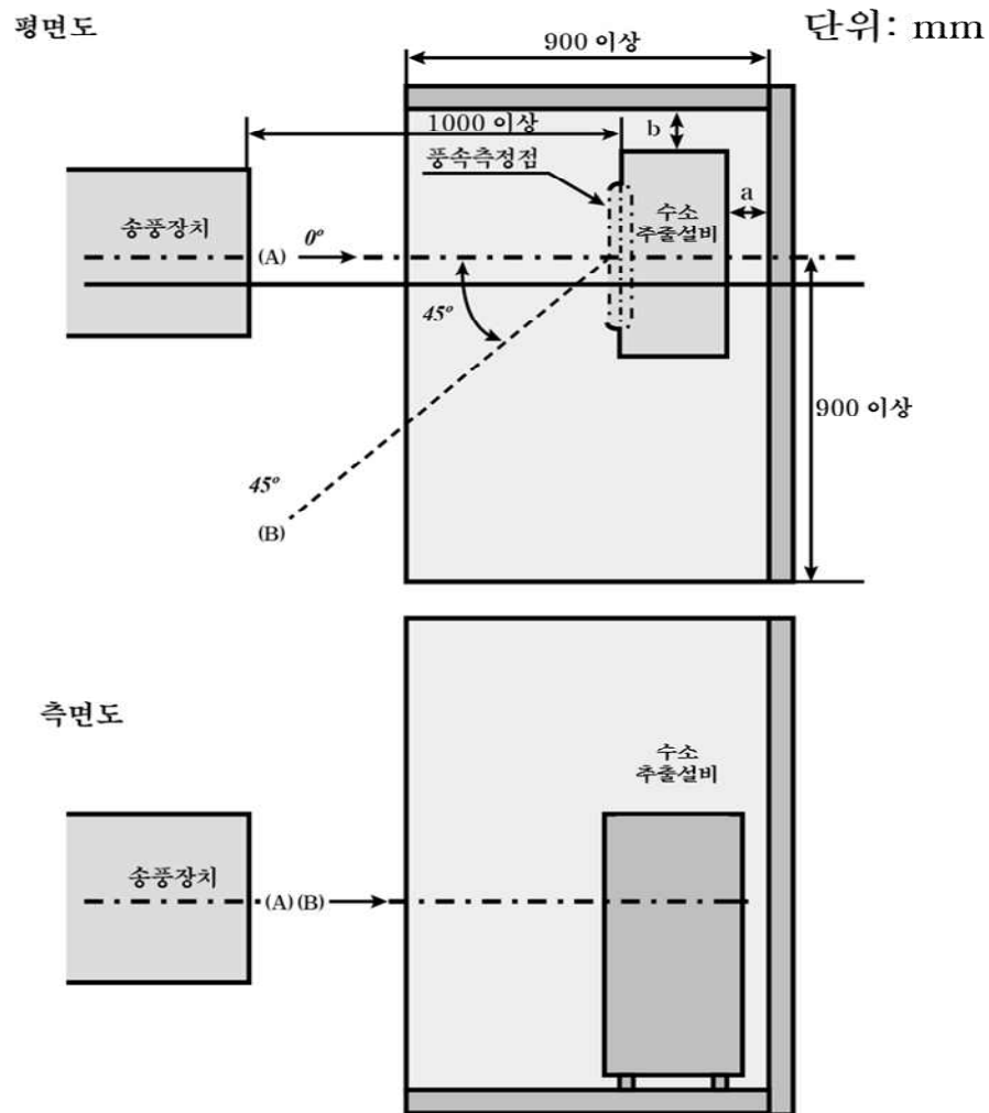
그림 C4.1 옥외식 유풀시험장치
