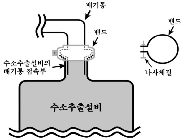
그림 3.2.8.2 “리프트업 연결부 예”
