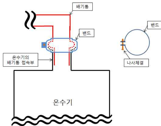
그림 3.2.13 리브 타입 연결부 예 <신설 17. 6. 2.>
