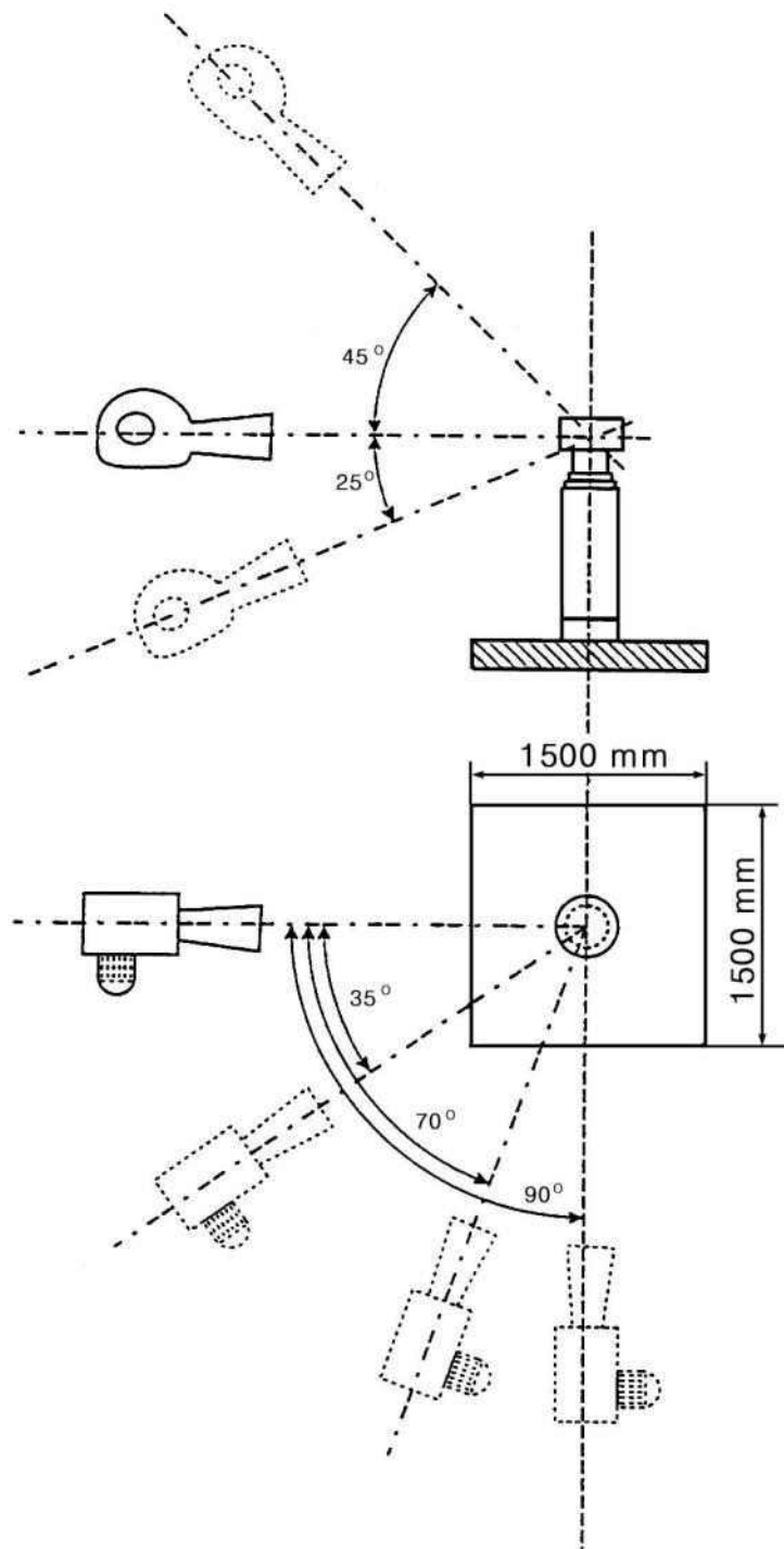
그림 E2. 지붕에 설치될 보일러 유풍 시험장비
