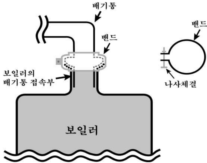
그림 3.2.10.1 리프트 타입 연결부 예 <신설 17. 6. 2.>
