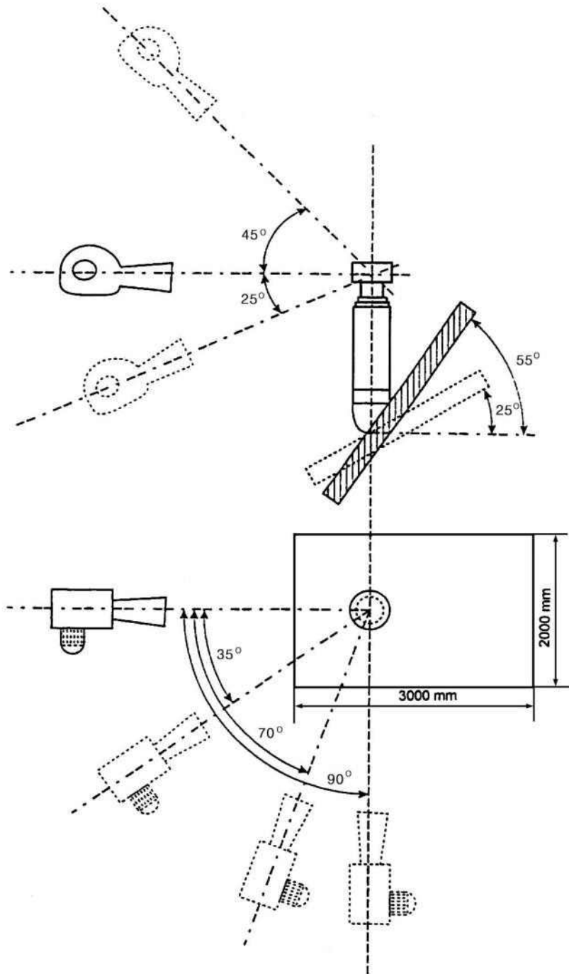
그림 E4. 지붕에 설치될 보일러 유평 시험장비
