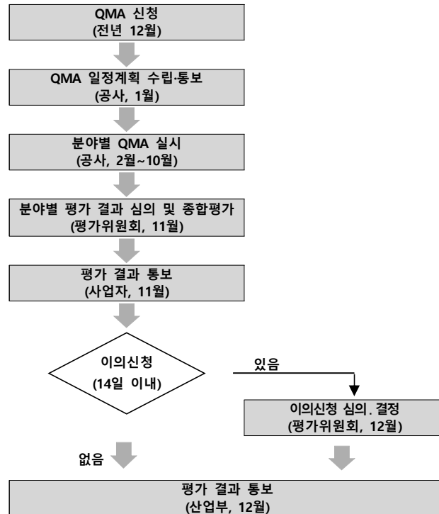
그림 7.2 안전관리수준평가(QMA) 프로세스
