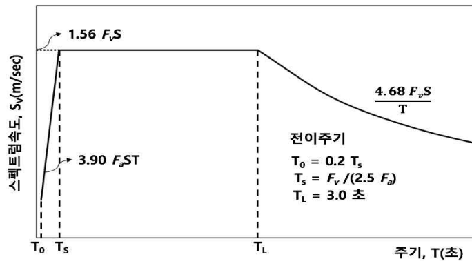
그림 2.5.6.1.2② 토사지반 수평지반운동의 속도 표준응답스펙트럼 <개정 22. 8. 30.>
