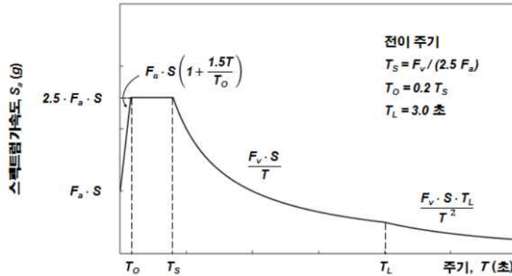
그림 2.5.6.1.2① 토사지반 수평지반운동의 가속도 표준응답스펙트럼 <개정 22. 8. 30.>
