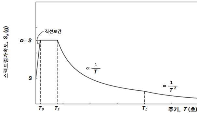
그림 2.5.6.1.1(1) 가속도 표준설계응답스펙트럼(암반지반) <개정 22. 8. 30.>
