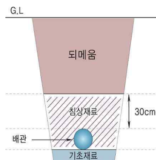
그림 2.5.7.5.5 배관의 매설방법
