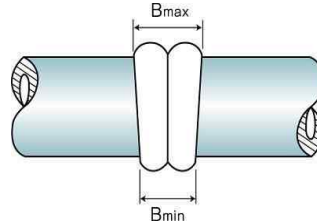
그림 2.5.4.2.2(1)② 용작이음부의 비드폭
