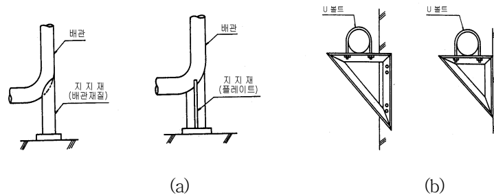
그림 F8.2 입상관 하부 견고한 지지의 예(자중 및 내진지지 겸용)
