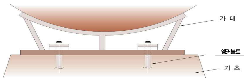
그림 2.2.3.4 앵커볼트의 고정방법 <개정 16.12.15>
