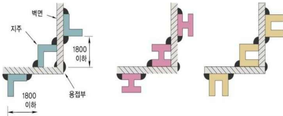
그림 2.9.2.3.4 지주의 설치방법
