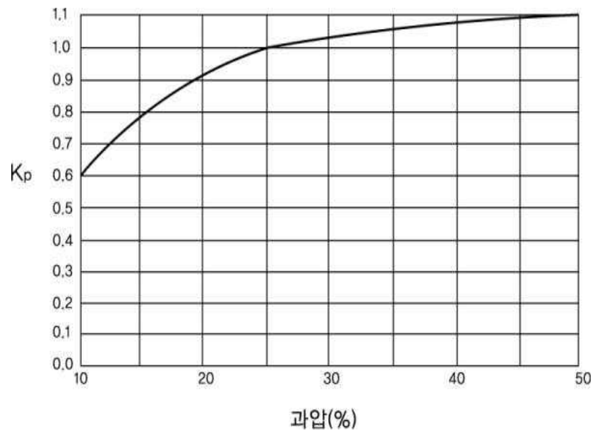
그림 2.8.1.4.2③ 과압보정계수
