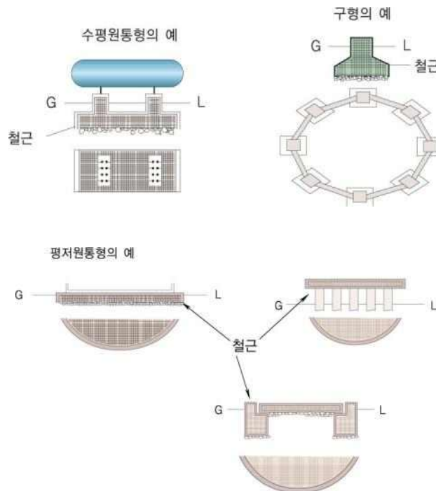
그림 2.2.2.3 저장탱크의 수평기초면
