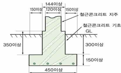
그림 2.9.2.1 철근콘크리트제 방호벽 설치예
