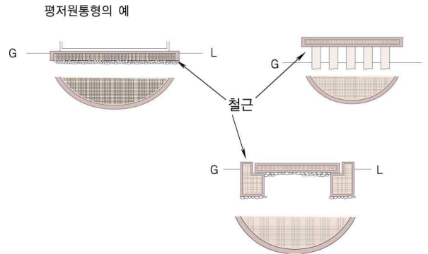
그림 2.2.2.3 저장탱크의 수평기초면
