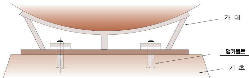
그림 2.2.3.4 앵커볼트의 고정방법 <개정 16.12.15>
