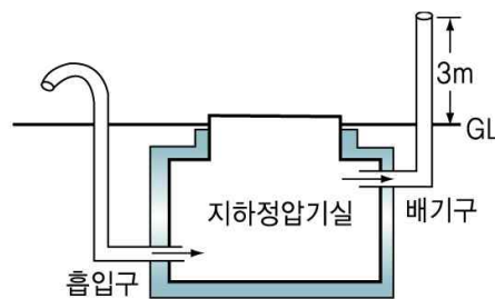
그림 27.4.1.3 공기보다 비중이 가벼운 가스를 사용하는 정압기가 지하에 설치된 경우 환기설비 설치 예
