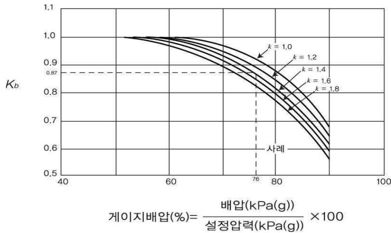
그림 2.7.1.4(2)③ conventional 안전밸브 배압조정계수
