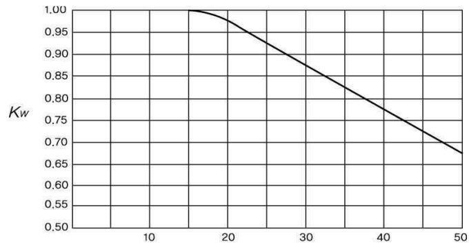
그림 2.7.1.4(2)⑤ 이음속계수
