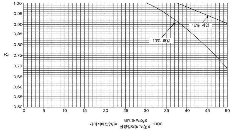
그림 2.7.1.4(2)② 벨런스 벨로즈형 안전밸브 배압보정계수
