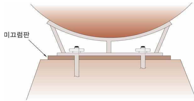
그림 2.2.3.5 미끄럼판의 설치 방법
