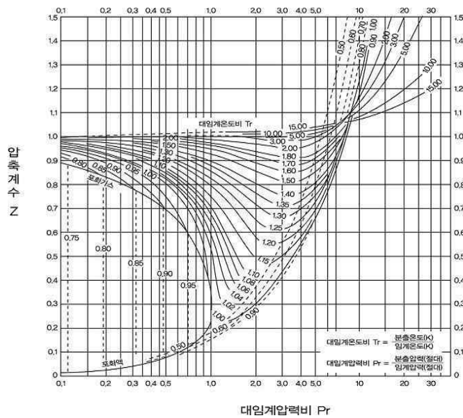
그림 2.7.1.4(2)④ 압축계수
