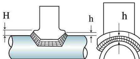
그림 2.5.5.2.7(1)④ 비드의 높이(h) 및 이음관 높이(H)
