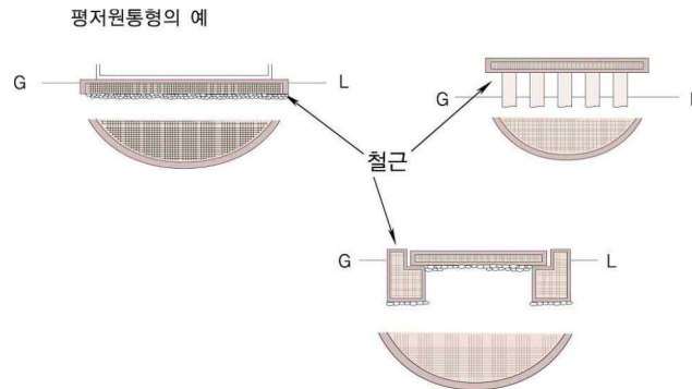
그림 2.2.2.4 저장탱크의 수평기초면
