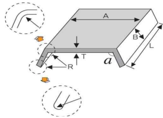
그림 2.5.8.2.2 보호판의 치수
