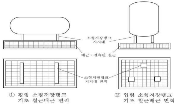
그림 2.3.3.6.3(3-3) 소형 저장탱크 일체형 철근콘크리트 기초의 철근 배근 예시
