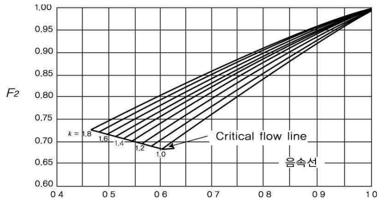
그림 2.7.1.4(2)⑤ 이음속계수
