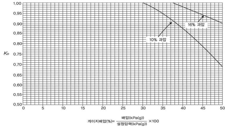
그림 2.7.1.4(2)② 밸런스 벨로즈형 안전밸브 배압보정계수
