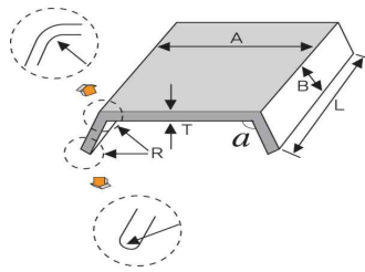
그림 2.5.8.2.2 보호판의 치수
