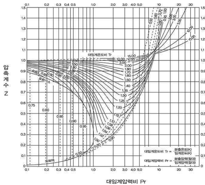
그림 2.7.1.4(2)④ 압축계수
