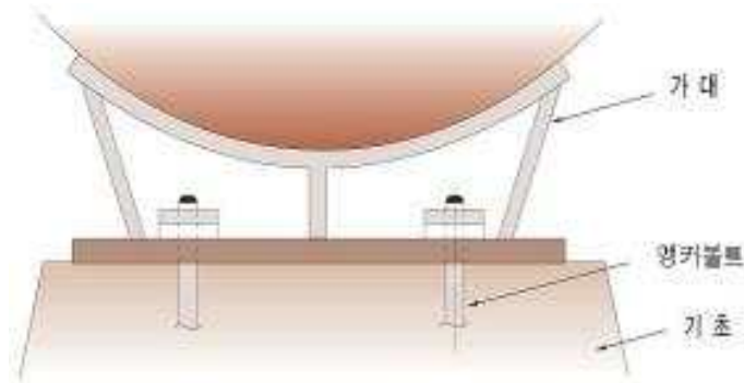
그림 2.2.3.4 앵커볼트의 고정 방법
