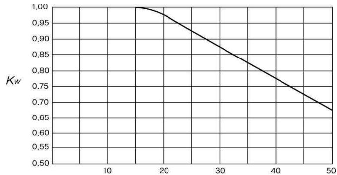
그림 2.7.1.4(2)⑤ 이음속계수
