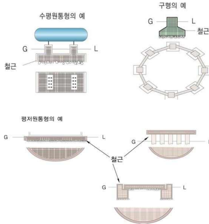
그림 2.2.2.3 저장탱크의 수평기초면
