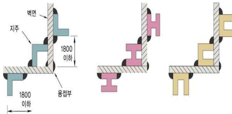
그림 2.8.2.3.4 지주의 설치방법
