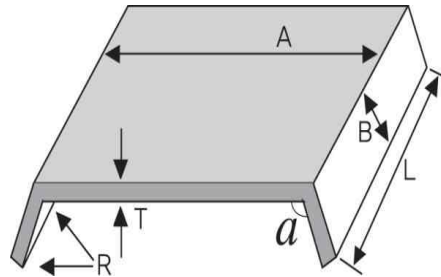
그림 2.5.8.2.3 보호판의 치수 측정
