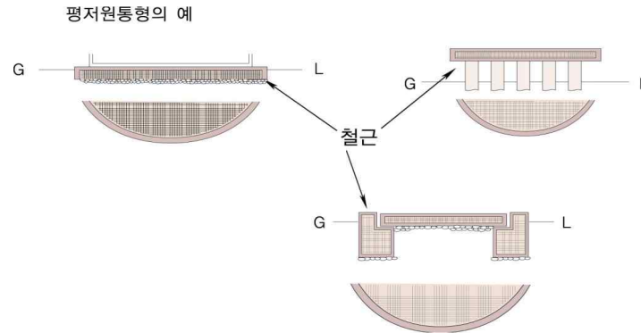
그림 2.2.2.3 저장탱크의 수평기초면
