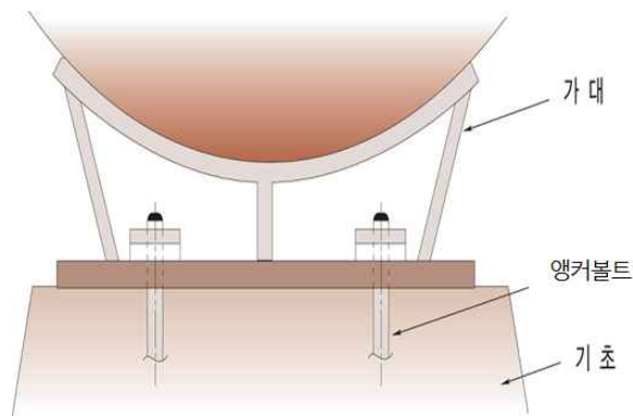
그림 2.2.3.4 앵커볼트의 고정방법 <개정 17.8.7>
