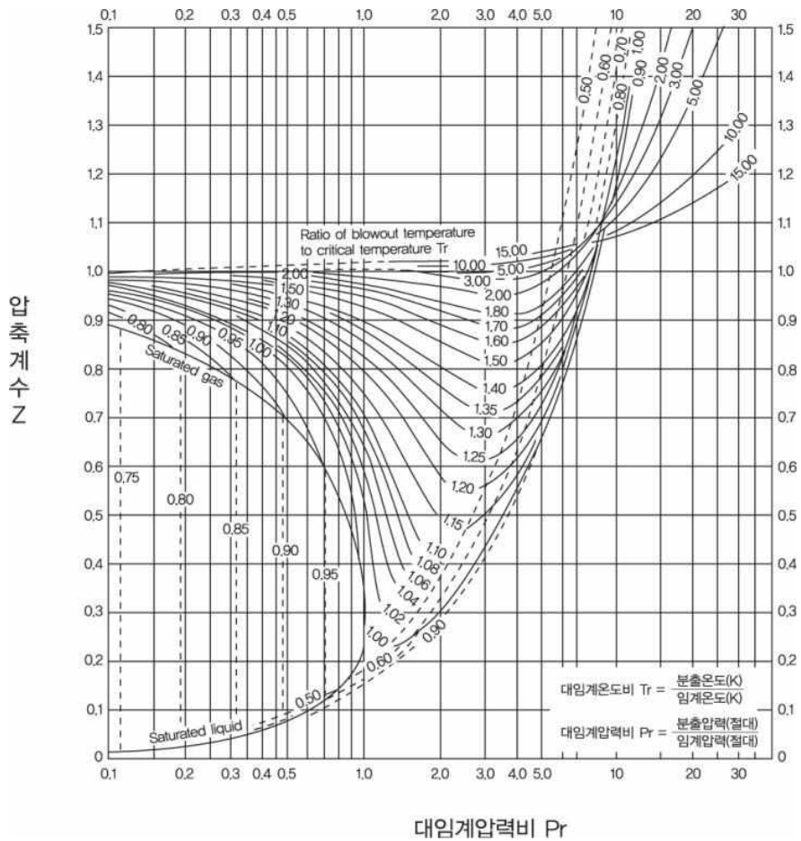
그림 2.6.1.4④ 압축계수
