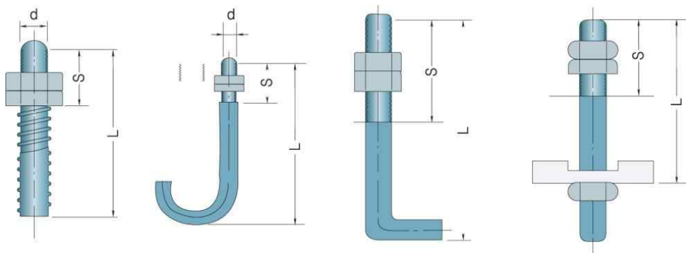
그림 2.2.3.3 앵커보울트의 치수표시
