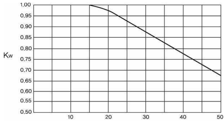
그림 2.6.1.4⑤ 아음속계수
