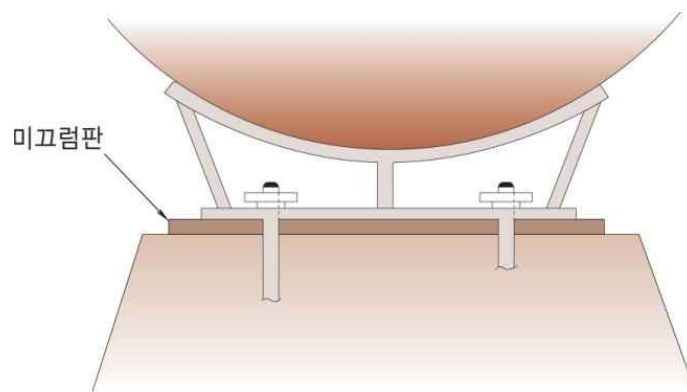
그림 2.2.3.5.3 미끄럼판의 설치방법
