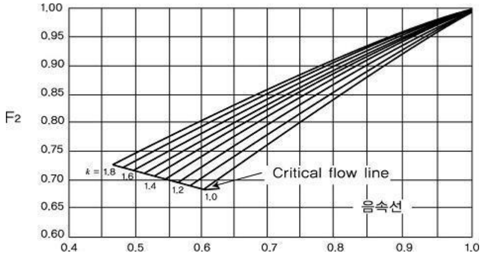
그림 2.6.1.4⑤ 아음속계수
