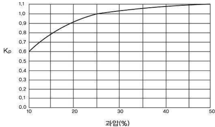
그림 2.6.1.4Ⓢ 과압보정계수
