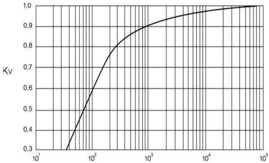
그림 2.6.1.4⑥ 밸런스 벨로우즈형 안전밸브 배압보정계수
