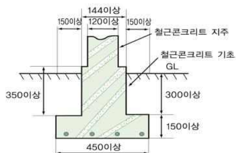
그림 2.7.2.2.2③ 철근콘크리트제 방호벽 설치예
