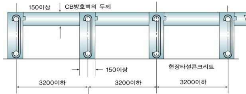
그림 2.7.2.3.2 보조벽의 배치
