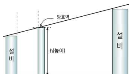
그림 2.7.2.1.3① 방호벽 설치 예(측면도)
