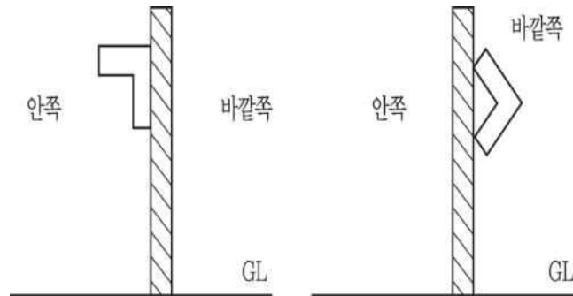
그림 2.7.2.4.2 강판제 방호벽의 앵글강 보강
