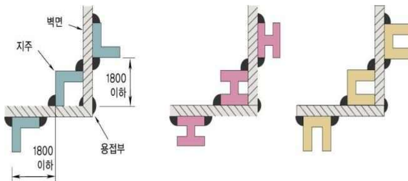
그림 2.7.2.4.4 지주의 설치방법
