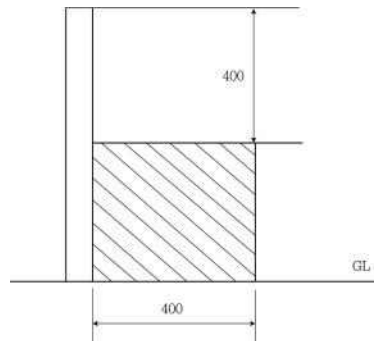
그림 2.7.2.3.3 보조벽의 높이
