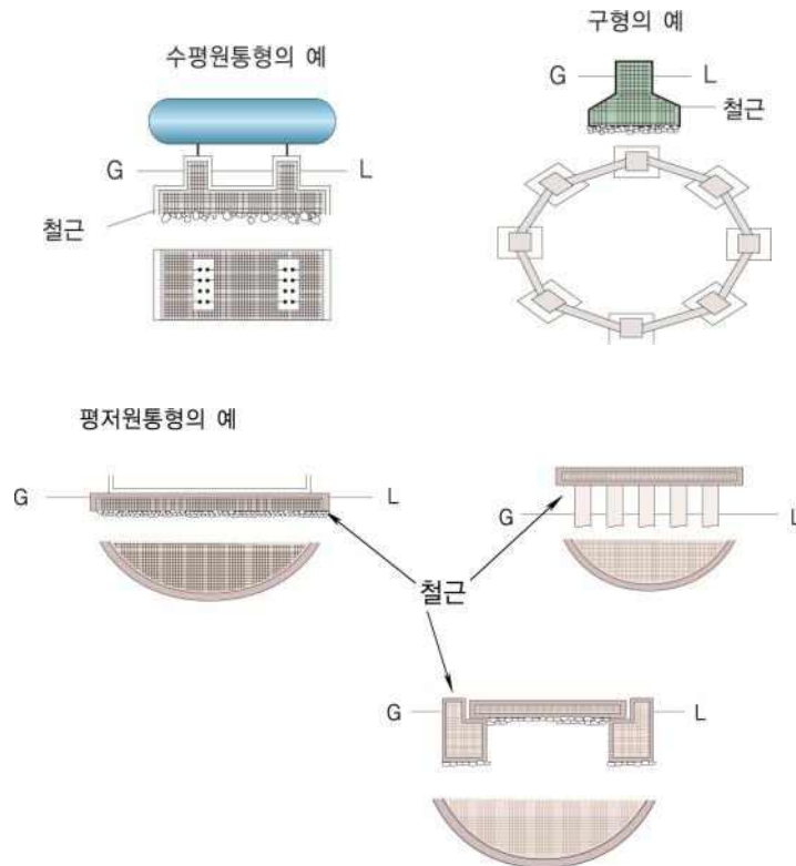
그림 2.2.2.3 저장탱크의 수평기초면
