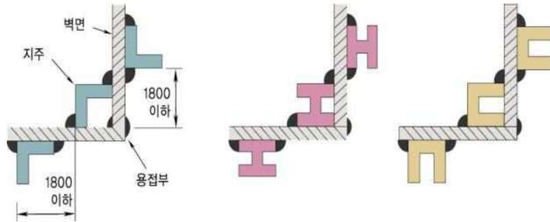
그림 2.7.2.4.4 지주의 설치방법
