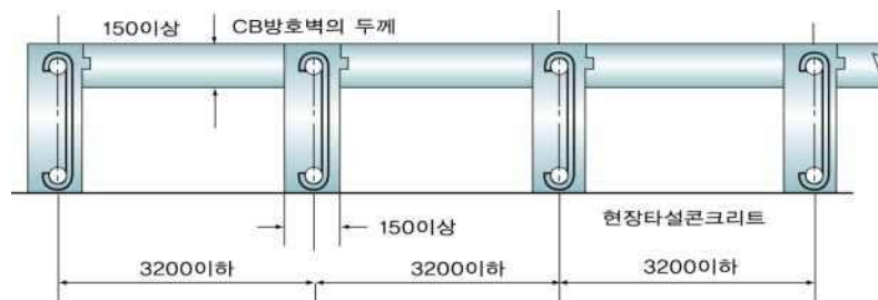
그림 2.7.2.3.2 보조벽의 배치
