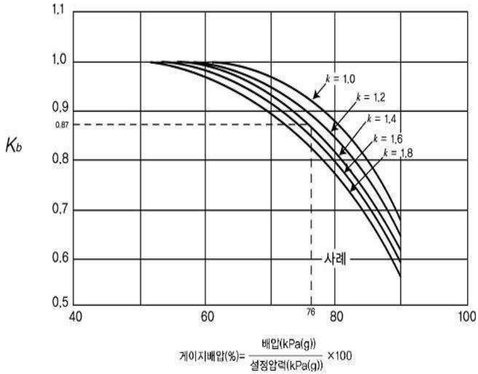
그림 2.6.1.4③ 일반형 (conventional) 안전밸브 배압조정계수
