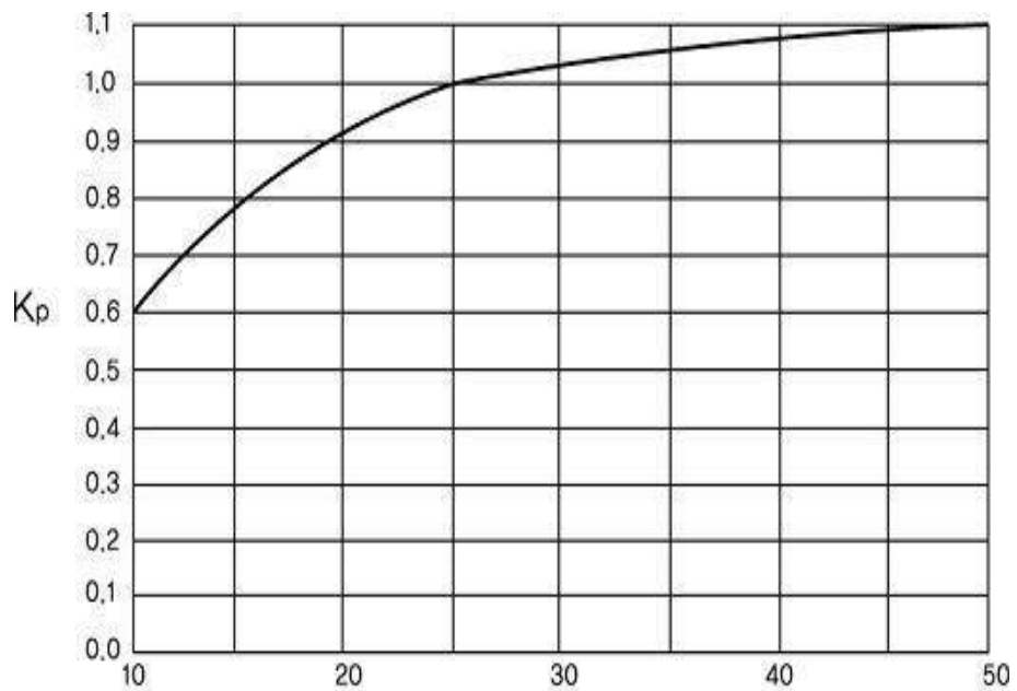
그림 2.6.1.4⑧ 과압보정계수
