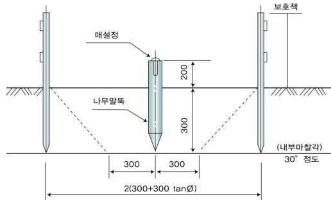
그림 3.1.2.1.2② 가벤치마크의 설정 예
