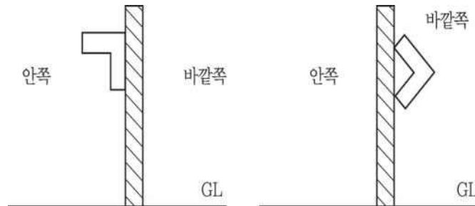
그림 2.7.2.3.2 강관제방호벽의 앵글강 보강
