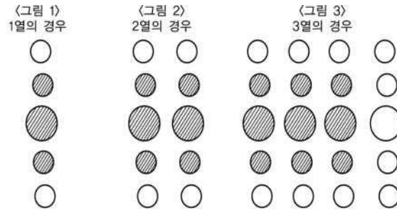
그림 2.9.9.1.3 온도상승방지설비 능력산정기준
