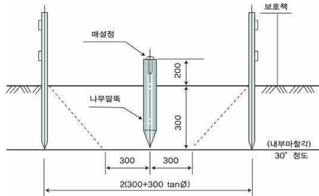
그림 3.1.2.1.2(2) 가벤치마크의 설정
