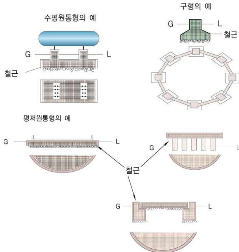
그림 2.2.2.3 저장탱크의 수평기초면
