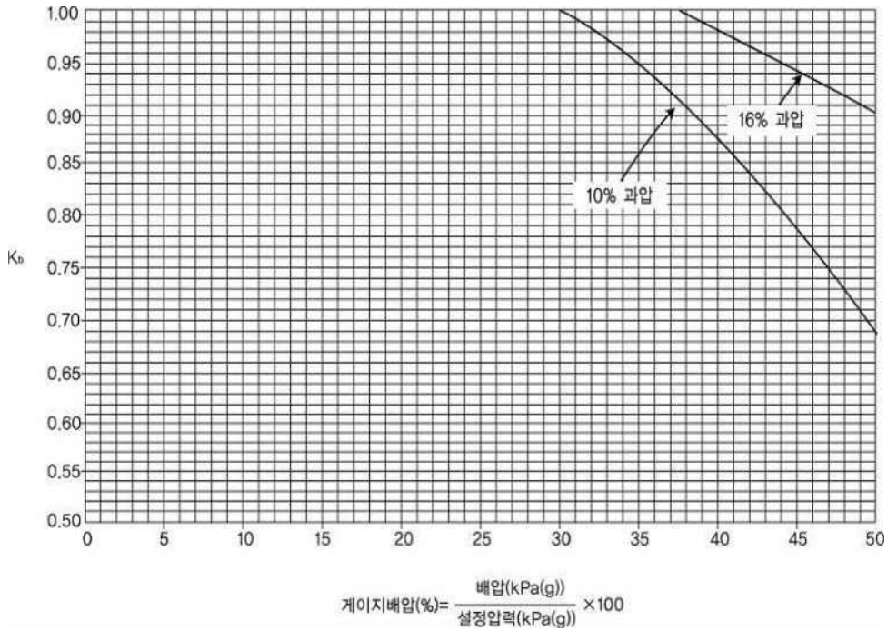
그림 2.6.1.4② 밸런스 벨로즈형 안전밸브 배압보정계수
