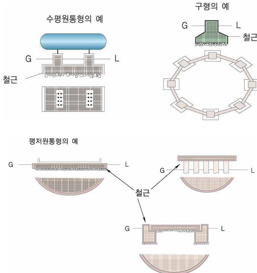
그림 2.2.2.3 저장탱크의 수평기초면
