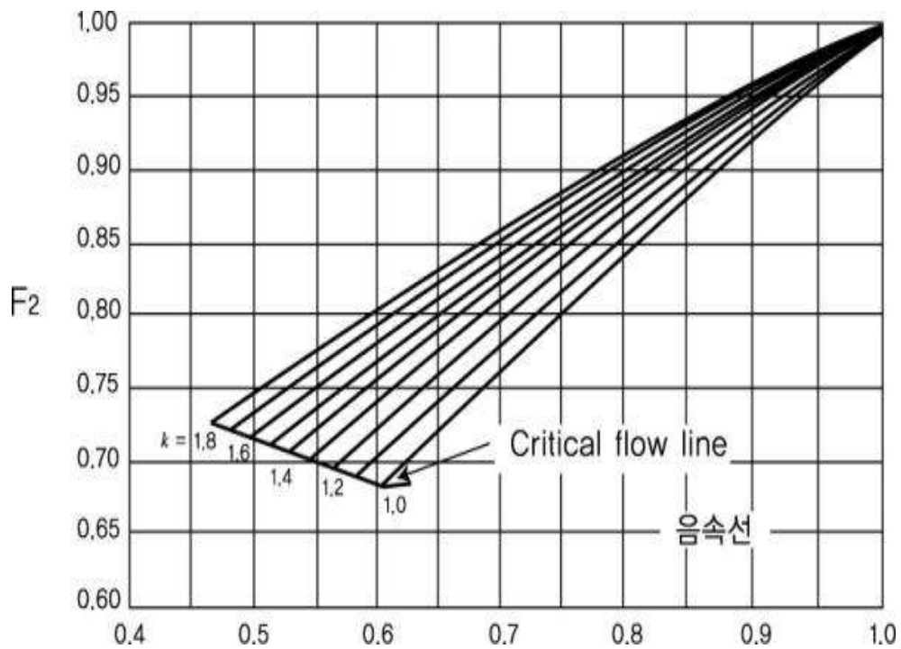
그림 2.6.1.4⑤ 이음속계수
