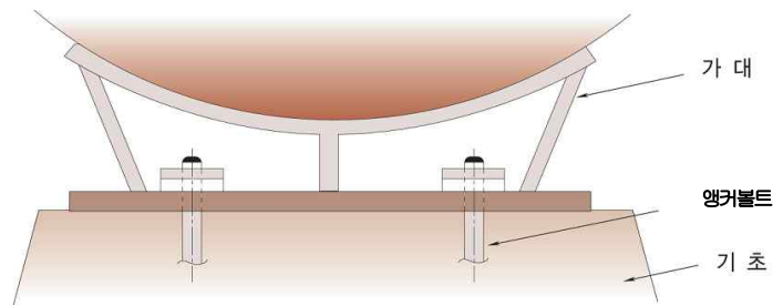
그림 2.2.3.4 앵커볼트의 고정방법 <개정 16.10.19>
