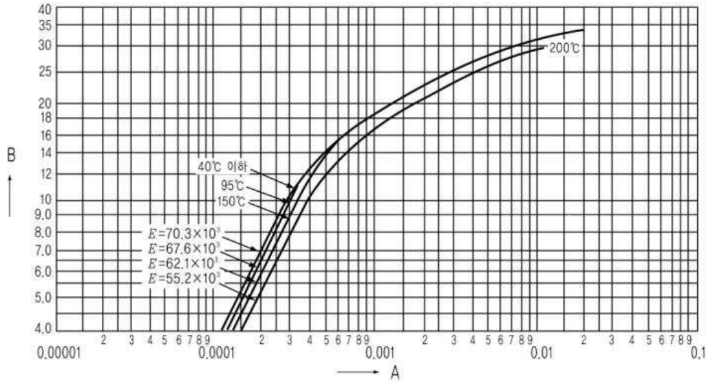
B-24 알루미늄 및 알루미늄합금(종류 5052, 5652, 질별 O, H12, H32, H112) (주) 이 그림을 적용하는 경우에는 규격 0.2% 내력이 규정되고 확인되어야 한다.
