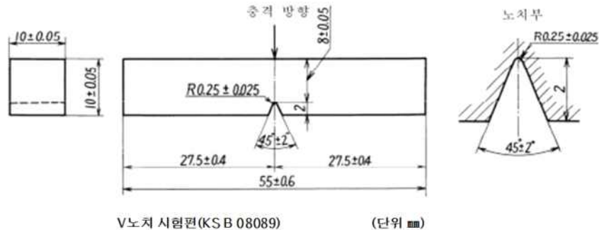
V노치 시험편(KS B 0809의 그림 1 V노치 시험편)
