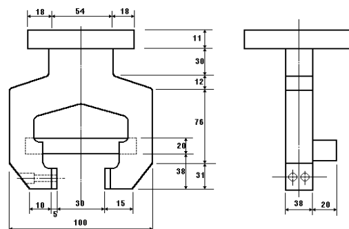
그림 3.11.2.2 밸브 부착 치구(예시)
