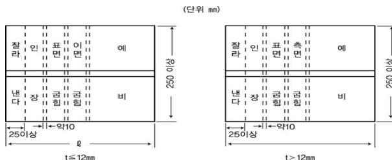
그림 4.4.2.2.1⑨ 시험판
