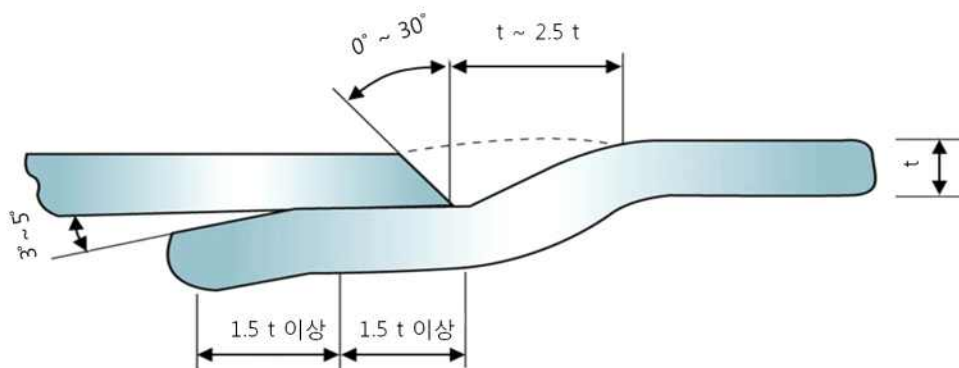
그림 2.1.1 joggle bending 용접 <개정 18.4.10>
