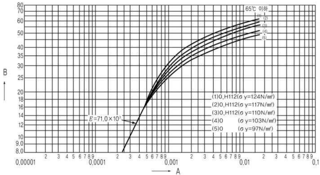
B-25 알루미늄 및 알루미늄합금(종류 5083 질별 O, H32, H112, H321, 종류 5086, 5154, 5254 질별 H32, H34)
