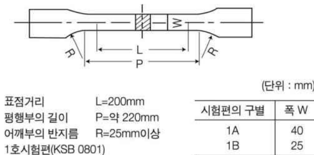
그림 4.4.2.2.1② 인장시험편(1호)
