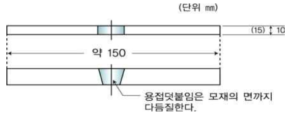
그림 4.4.2.2.1⑫ 측면굽힘 시험편
