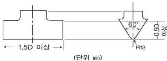
그림 4.4.2.2.1④ 췌기모양
