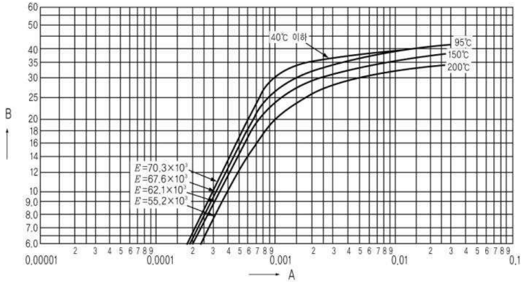
B-28 알루미늄 및 알루미늄합금 (종류 5454 질별 O, H112 종류 2014 질별 T4, T6)
