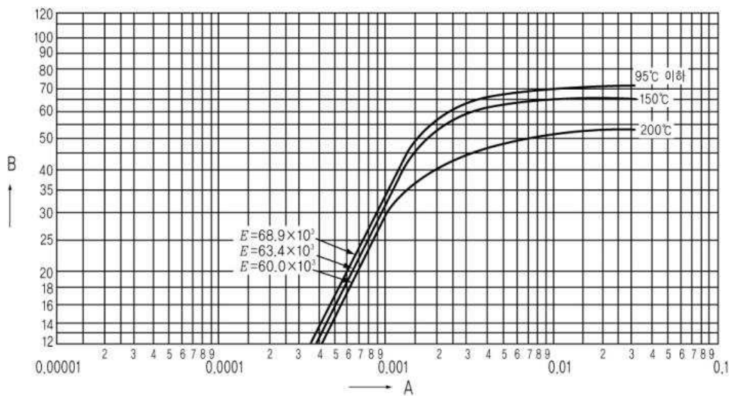
B-29 알루미늄 및 알루미늄합금(종류 6061 질별 T6, T651) (주) 이 그림은 5356 및 5556의 용가재를 사용하여 용접하는 경우에는 모든 모재 두께에 적용하고, 4043 및 5554의 용가재를 사용하여 용접하는 경우에는 모재 두께 9.5mm 이하에 적용한다.
