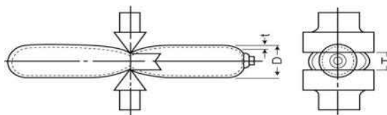
그림 4.4.2.2.1④ 췌기모양
