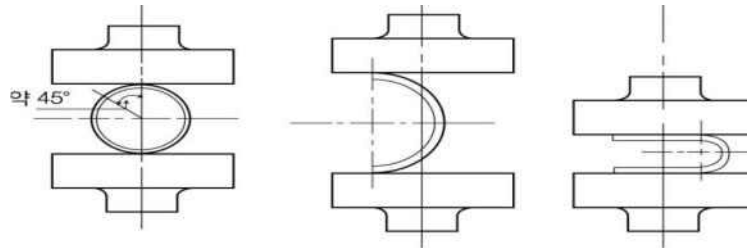
그림 4.4.2.2.1⑥ 중앙부에 길이이음매가 있는 시료의 위치
