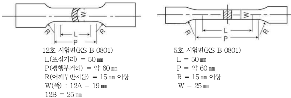
그림 4.4.2.2.1① 인장시험편 (5호, 12호)
