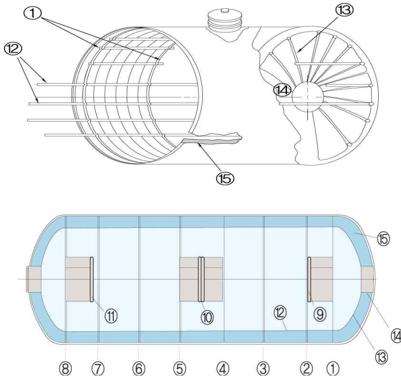
전체조립도
