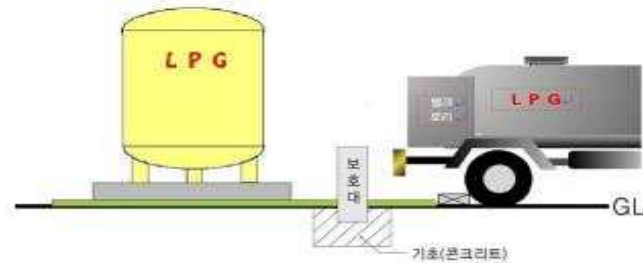
그림 2.3.3.4(6-7) 철근콘크리트 보호대 설치방법 예시
