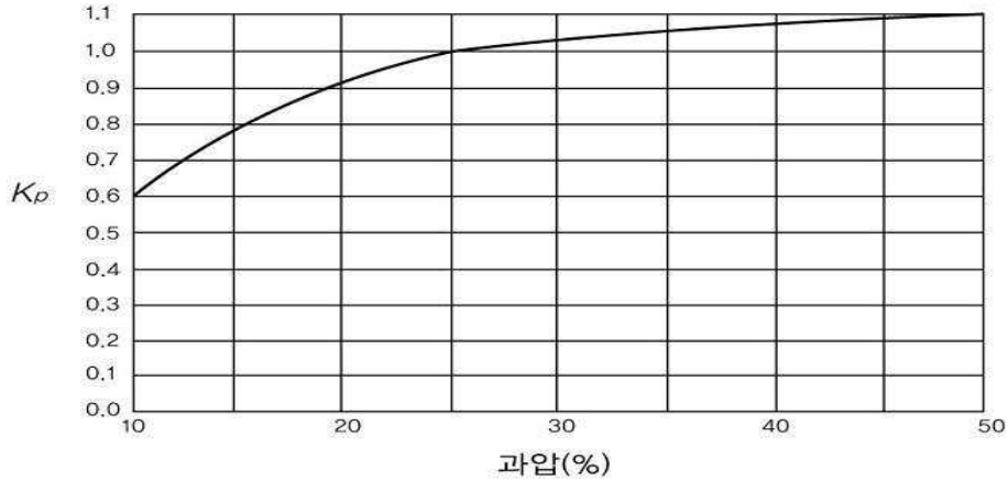
그림 2.8.1.4.1(2) ⑧ 과압보정계수
