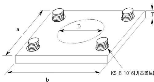
그림 2.3.3.4(6-4-2) 강관계 보호대의 받침대 설치 방법
