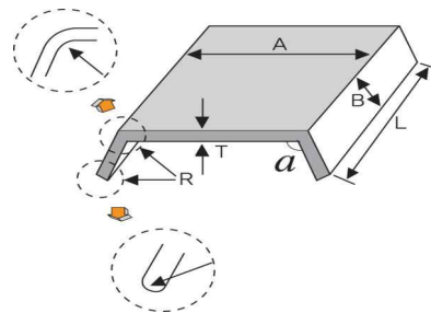
그림 2.5.7.5.3 보호관의 치수
