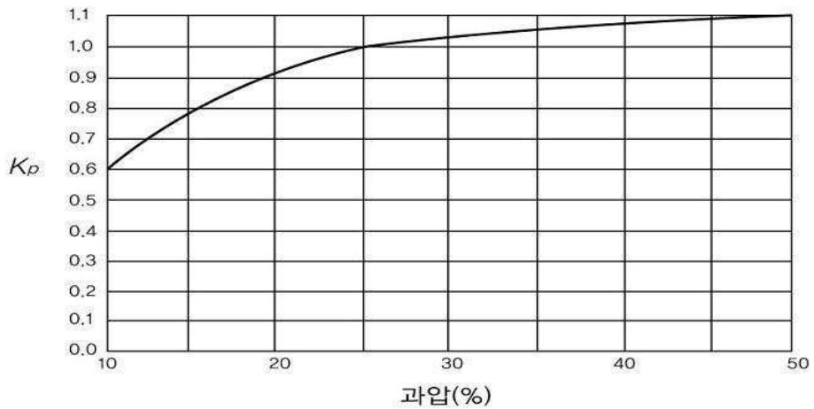
그림 2.8.1.4.1(2) ⑧ 과압보정계수
