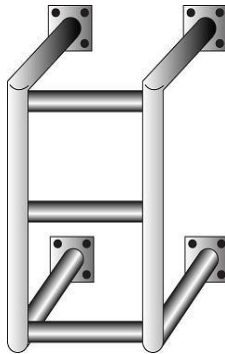
그림 2.5.7.6.9(2)② “ㄷ”형태로 가공한 강관제 구조물에 의한 방호조치
