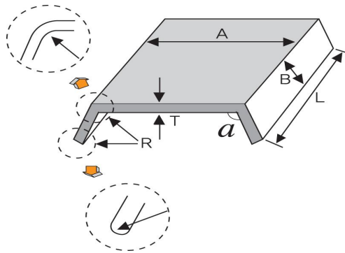
그림 2.5.7.5.3 보호관의 치수
