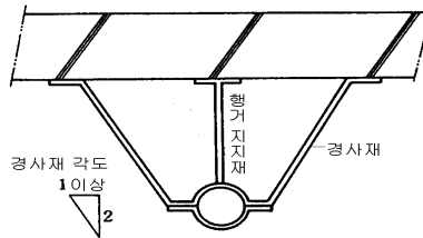
(c) 트러스지지
