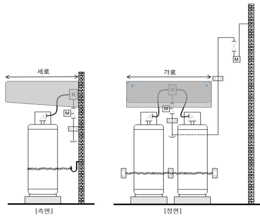
그림 2.3.2.1③ 용기 및 용기부속품 보호관 설치 예시
