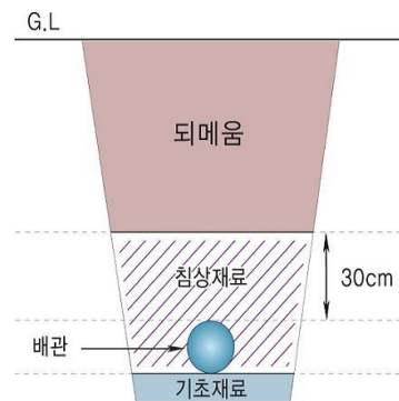
그림 2.5.7.5.5) 배관의 매설방법
