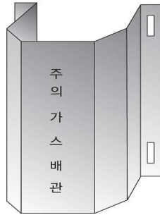
그림 2.5.7.6.9(2)① “ㄷ”형태로 가공한 철판제 방호구조물에 의한 방호조치
