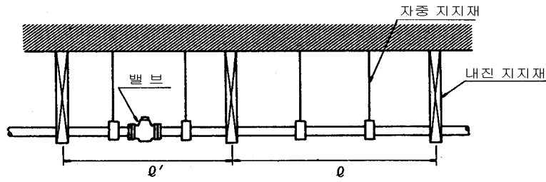
그림 E9.3 밸브 설치 시 지지의 예
