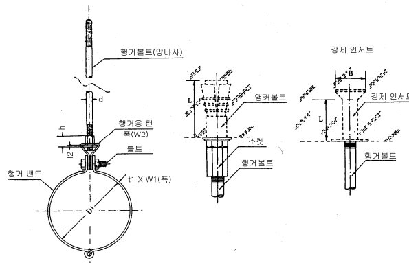
그림 E9.5② 행지관 자중지지구의 예(상세도)
