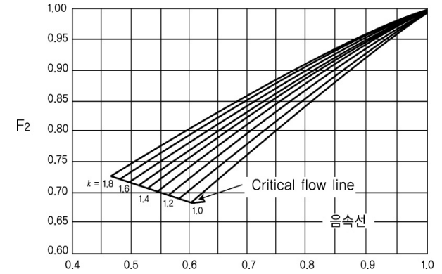
2.8.1.4.1⑤ 아음속계수
