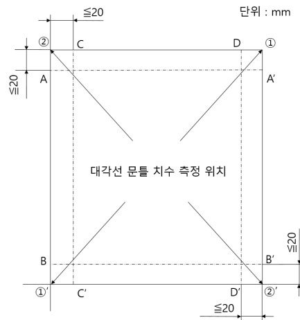
그림 3.2 방호문의 치수측정 위치
