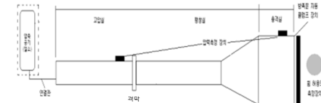
그림 4.2 폭발압력저항시험장치 구성도
