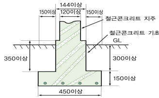
그림 2.9.2.1 철근콘크리트제 방호벽 설치예
