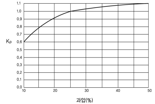
그림 2.8.1.4.2③ 과압보정계수
