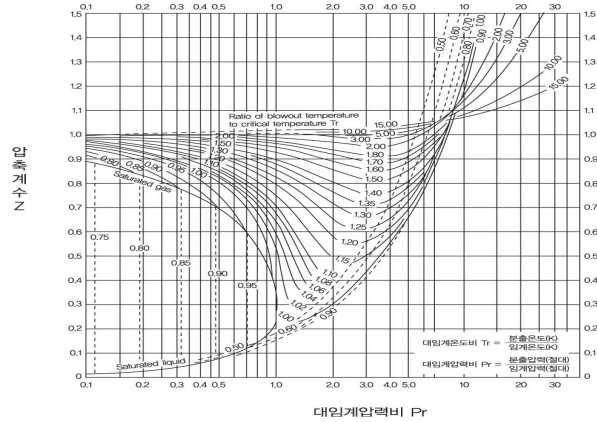
그림 2.8.1.4.1③ Conventional 안전밸브 배압조정계수
