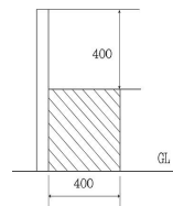
그림 2.9.2.2.3 보조벽의 높이
