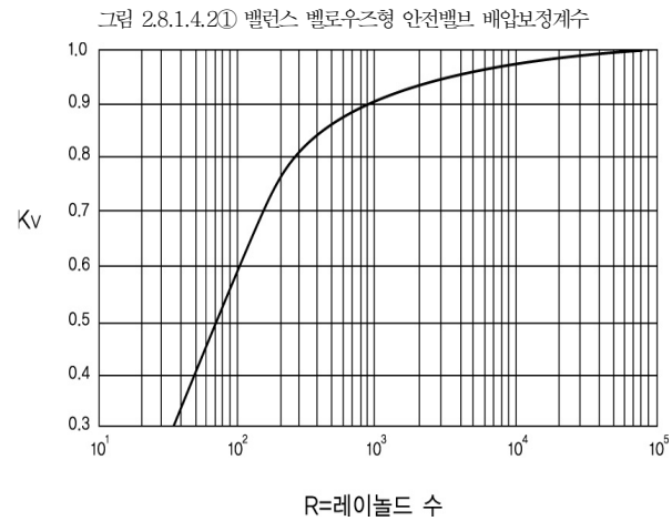
그림 2.8.1.4.2② 점도로 인한 용량보정계수
