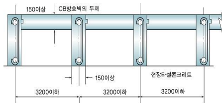
그림 2.9.2.2.2 보조벽의 배치
