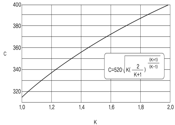
그림 2.8.1.4.1① 열용량비 k=C_p/C_v
