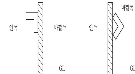
그림 2.9.2.3.2 강판제방호벽의 앵글강 보강
