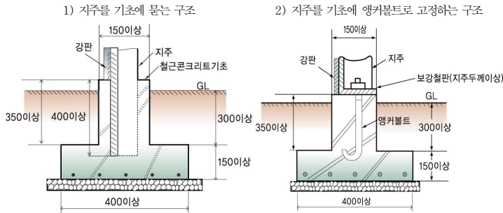
그림 2.9.2.3.6 강판제 방호벽의 고정방법 예
