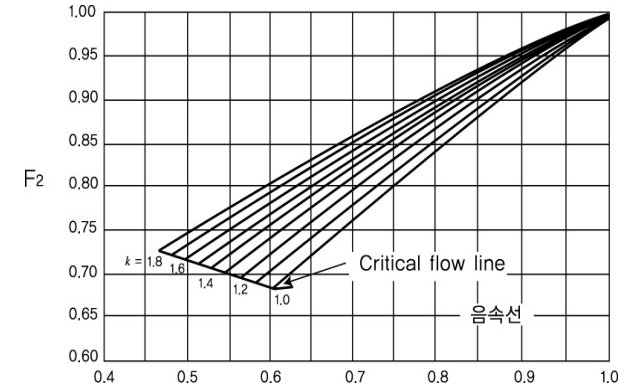
2.8.1.4.1⑤ 아음속계수
