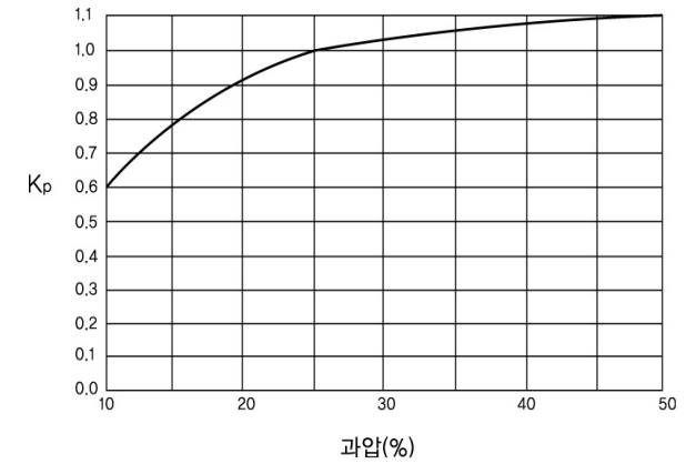
그림 2.8.1.4.2③ 과압보정계수
