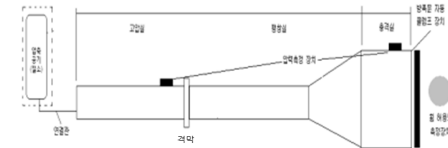
그림 4.2 폭발압력저항시험장치 구성도
