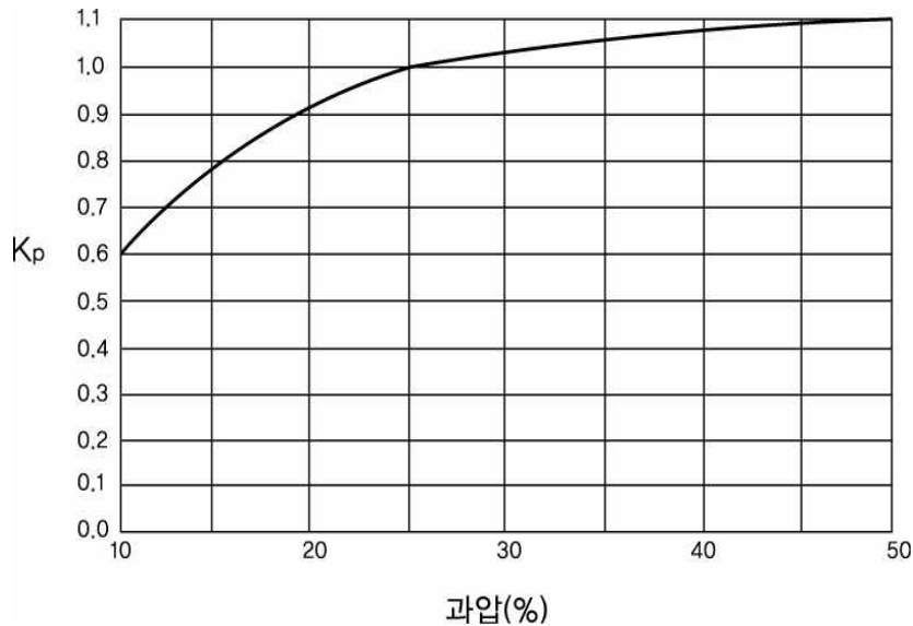
그림 2.8.1.4.2③ 과압보정계수
