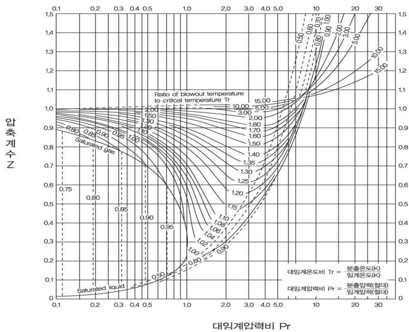
그림 2.8.1.4.1④ 압축계수
