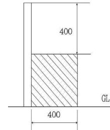
그림 2.9.2.2.3 보조벽의 높이
