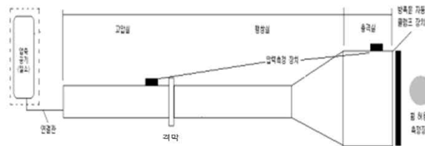
그림 4.2 폭발압력저항시험장치 구성도
