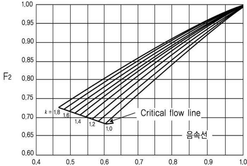
그림 2.8.1.4.1④ 압축계수
