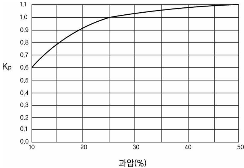
그림 2.8.1.4.2② 점도로 인한 용량보정계수
