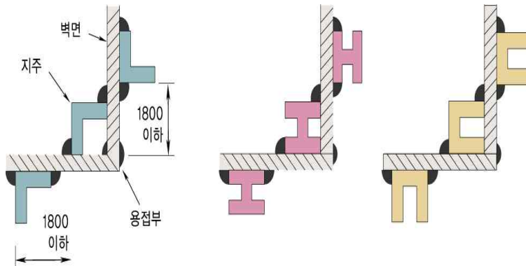
그림 2.9.2.3.4 지주의 설치방법
