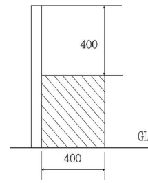
그림 2.9.2.2.3 보조벽의 높이
