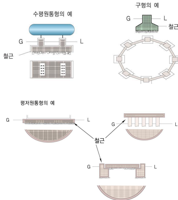
그림 2.2.2.3 저장탱크의 수평기초면
