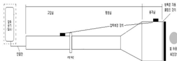
그림 4.2 폭발압력저항시험장치 구성도
