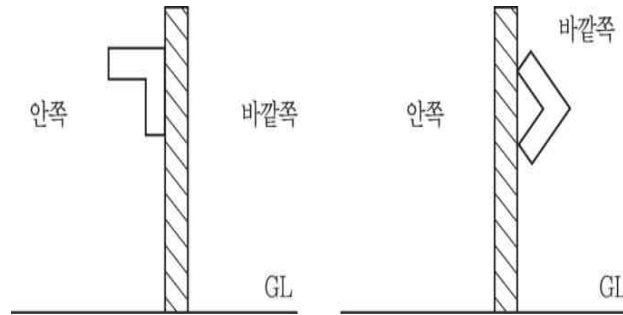
그림 2.9.2.3.2 강관제방호벽의 앵글강 보강
