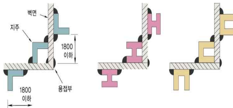
그림 2.9.2.3.4 지주의 설치방법
