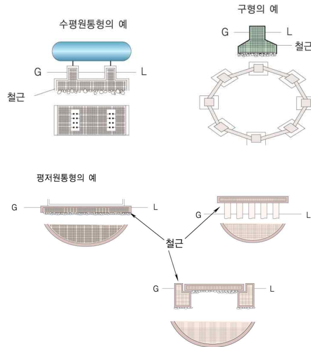
그림 2.2.2.3 저장탱크의 수평기초면
