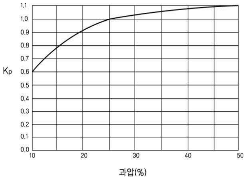
그림 2.8.1.4.2③ 과압보정계수
