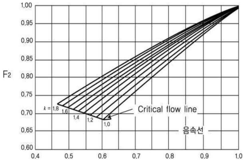
2.8.1.4.1⑤ 아음속계수
