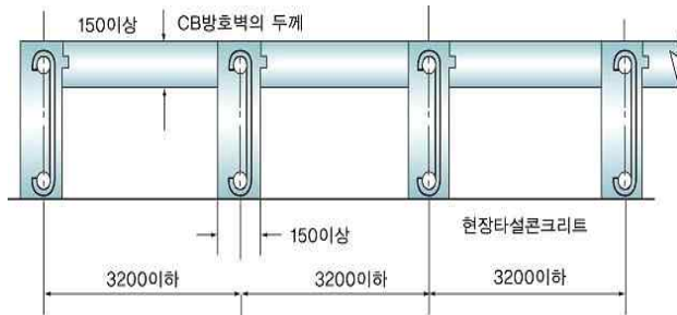
그림 2.8.2.2.2 보조벽의 배치
